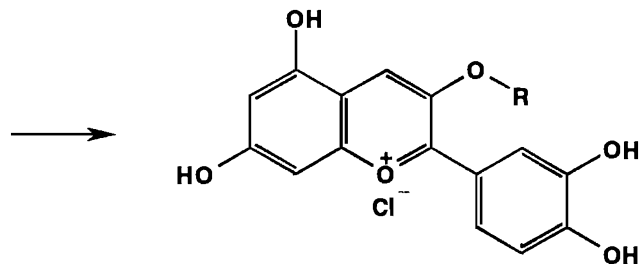
цианин хлорид (пирилиевая соль)
