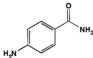
амид p -аминобензойной кислоты
