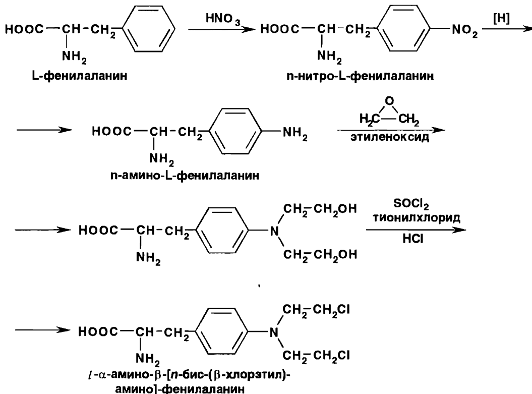
26.1. Свойства сарколизина и мелфалана
