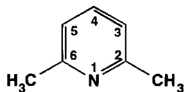
2,6-диметилпиридин (2,6-лутидин)
