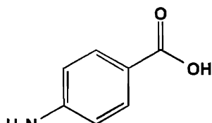
p -аминобензойная кислота
