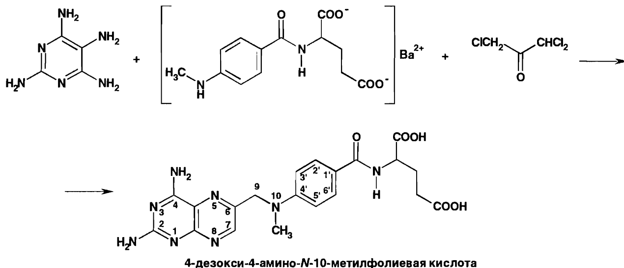
68.2. Свойства метотрексата
