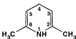
1,4-дигидро- 2,6-диметил- пиридин
