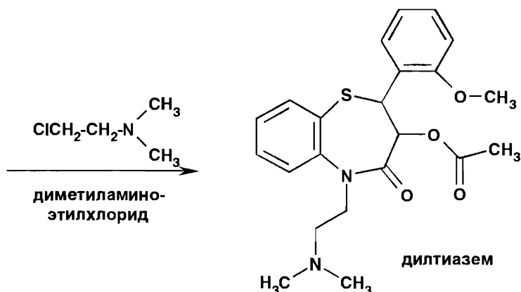
71.6. Свойства дилтиазема гидрохлорида
