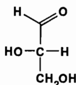
l -глицериновый альдегид
