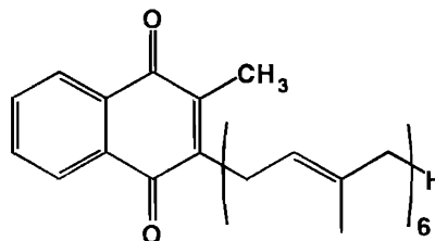
менахинон-6 или витамин K_2(30) (2-метил-3-дифарнезил-1,4- -диоксонафталин)
