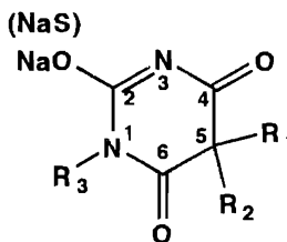
натриевые соли барбитуратов
