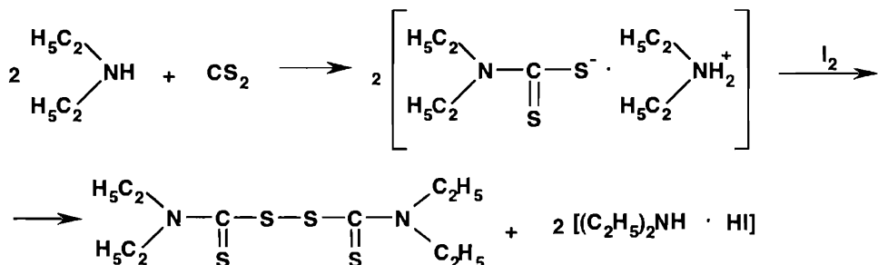
28.1. Свойства дисульфирама
