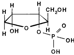
\alpha -D-рибофуранозы фосфат
