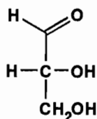
d -глицериновый альдегид
