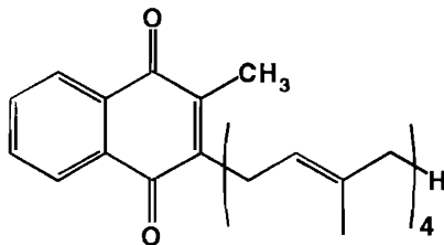
менахинон-4 или витамин K_2(20) (2-метил-3-дигеранил-1,4- -диоксонафталин)
