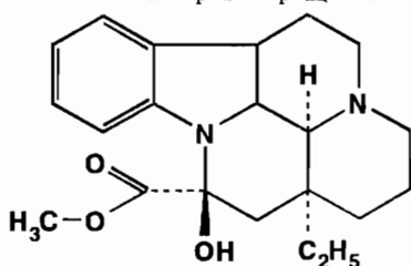
девинкан (метилевый эфир винкаминовой кислоты)
