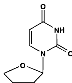
N' -(2-фуранидил) урацил
