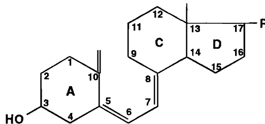
общая формула кальциферолов
